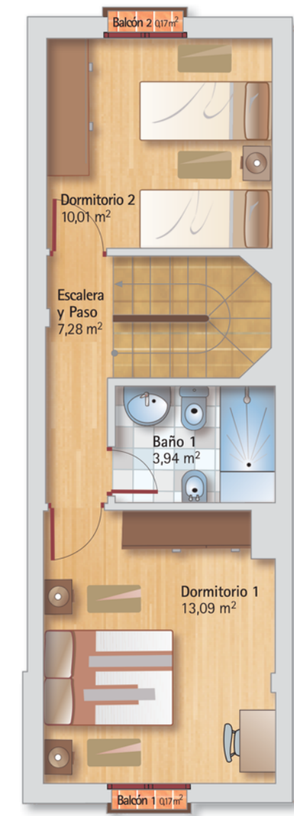
Planta 2
